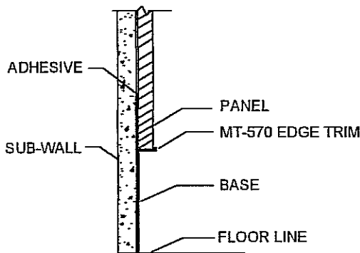
Edge Trim
